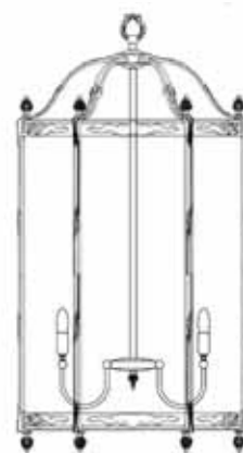
Art1881/G H 120 cm Ø 63cm 8x E27 x 60W
