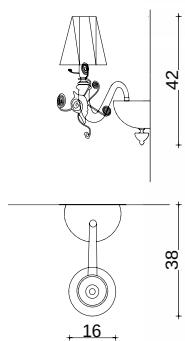
Art. 1631/A1 H 42 cm Sp 38 cm PØ 16 cm 1 x E14 x 40W
