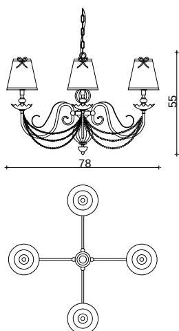
ART. 1794/CH4 H 55cm ø78cm Pø 16 cm 4xE14x40W
