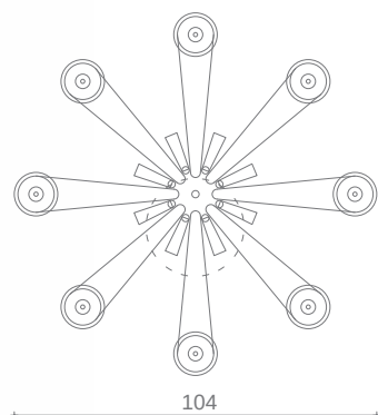
Art. 1770/CH8 H 90cm Ø 104 cm PØ 12 cm 8 x E14 x 40W
