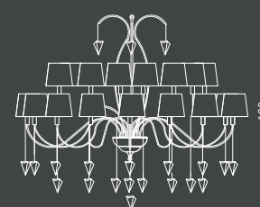
Art. 1740/CH12/KR/V2 H 80 cm Ø 86cm Pd 14cm 12 x E14 x 40w
