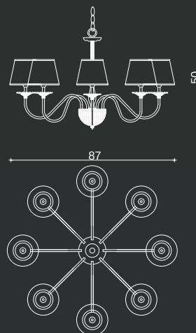
Art. 1460/CH8 H 50 cm ø 87 cm Pø 16 cm 8 x E14 x 40W
