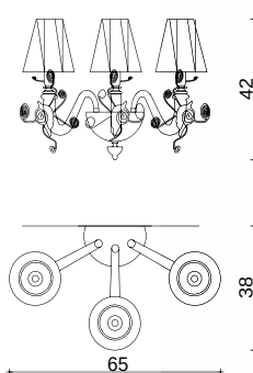
Art. 1631/A3 H 42 cm L 65cm Sp 38 cm PØ 16 cm 3 x E14 x 40W
