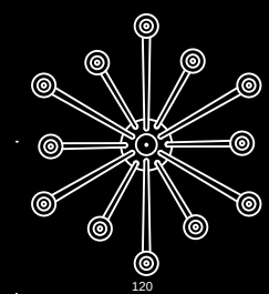
Art.1761 CH12 H 150cm Ø 120cm 12x E14 x 40W
