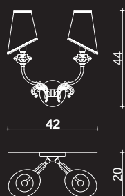
ART. 1774/A2 H 44 cm ø 42 cm Pø 14 cm 2 x E14 x 40W
