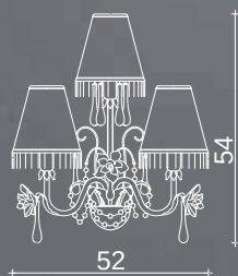
Art. 1627/A3 H 54 cm ø 52 cm Sp 15cm Pø 14 cm 3 x E14 x 40W
