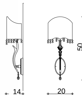
ART. 1689/A1/V2 H50cm L20cm Sp 14cm 1x E14 x 40W
