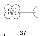
ART. 1689/A1/V1 H 45cm Sp37cm P Ø 18cm 1x E14 x 40W
