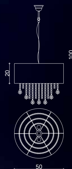
Art. 1386/CH2 H100 cm Pø 50cm 2xE27x60W
