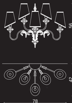
ART. 1774/A5 H 56 cm ø 78 cm Sp 42cm Pø 14 cm 5 x E14 x 40W
