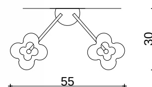
ART. 1689/A2 H 45cm L 55cm Sp 30cm PØ 18 cm 2x E14 x 40W
