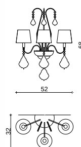
Art. 1742/A3/KR H 68 cm ø 52 cm Pø 14 cm 3 x E14 x 40W
