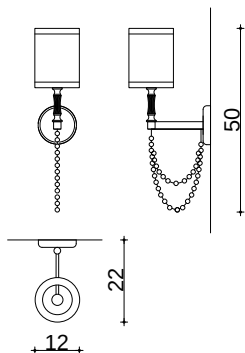
Art. 1703/A1/LU/TR H 50 cm Sp 22cm Pø 12 cm 1x E14 x 40W
