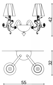
Art. 1631/A2 H 42 cm L 55cm Sp 32 cm PØ 16 cm 2 x E14 x 40W
