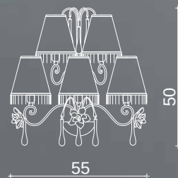
Art. 1627/A5 H 50 cm ø 55 cm Sp 15cm Pø 14 cm 5 x E14 x 40W
