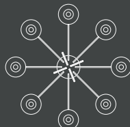
Art. 1740/CH8/V1 H 80 cm ø 86 cm Pø 14 cm 8 x E14 x 40W
