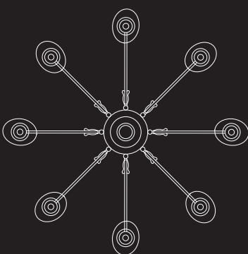
ART. 1774/CH8 H 66 cm ø 110 cm Pø 14 cm 8 x E14 x 40W
