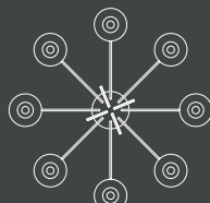
Art. 1710/CH8/KR/RS/V1 H 80 cm ø 86 cm Pø 14 cm 8 x E14 x 40W
