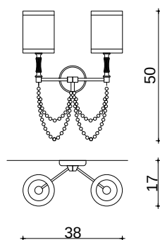
Art. 1703/A2/LU/TR H 50 cm L 38 cm SP 17cm Pø 12 cm 2 x E14 x 40W
