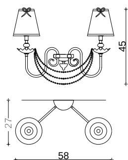
ART. 1794/A2 H 45cm Sp 27cm Pø 16 cm 2xE14x40W
