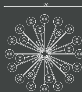
Art. 1740/CH24 H 100 cm ø 120 cm Pø 14 cm 24 x E14 x 40W
