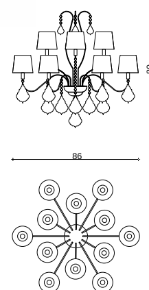
Art. 1742/CH12/KR/V2 H 80 cm ø 86 cm Pø 14 cm 8 x E14 x 40W
