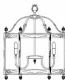
Art1881/P H 76 cm Ø 63cm 6 x E27 x 60W
