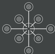
Art. 1740/CH8/KR/V2 H 75 cm ø 86 cm Pø 14 cm 8 x E14 x 40W
