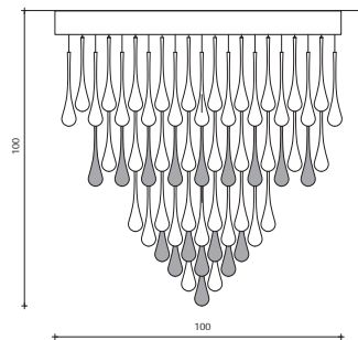
Art. 1615 H 100 cm ø 100 cm 16 x E14 X 40W
