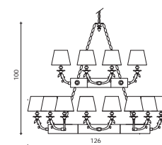
Art. 1543/CH24 H 100 cm ø 126 cm Pø 16 cm 24 x E14 X 40W
