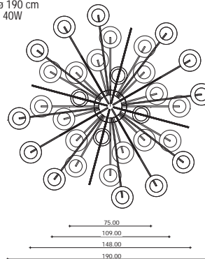
Art. 1451/CH32 H 185 cm ø 190 cm 32 x E14 X 40W
