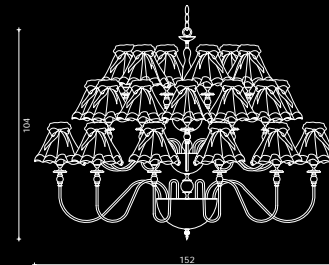
Art. 1580/CH30 H 104 cm ø 152 cm Pø 26 cm 30 x E14 X 40W
