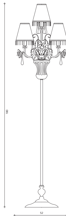
Art. 1627/FL H 180 cm ø 52 cm Pø 14 cm 5 x E14 X 25W
