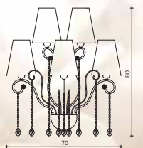
Art. 1630/A5 H 80 cm ø 70 cm Pø 18 cm 5 x E14 X 40W Applique
