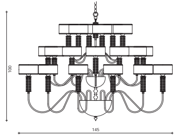
Art. 1423/CH30 H 100 cm ø 145 cm Pø 18 cm 30 x E14 X 40W
