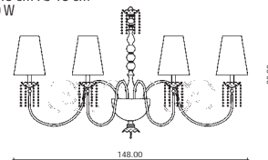
Art. 1507/CH8 H 82 cm ø 148 cm Pø 18 cm 8 x E14 X 40W
