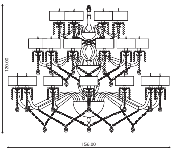
Art. 1352/CH30 H 120 cm ø 156 cm Pø 18 cm 30 x E14 X 40W
