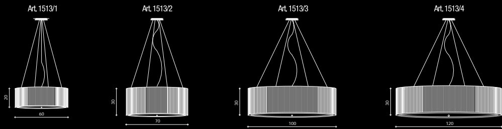
Art. 1513 H 44 cm Pø 100 cm 4 x E27 x 60W
