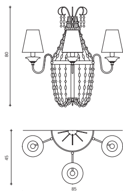
Art. 1380/A3 H 80 cm ø 85 cm Pø 18 cm 3 x E14 X 40W
