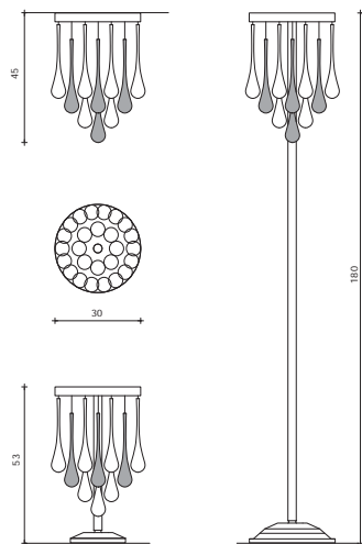
Art. 1359/TA H 53 cm ø 30 cm 3 x E14 X 40W
