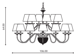
Art. 1447/CH18 H 64 cm ø 106 cm Po 16 cm 18 x E14 X 40W
