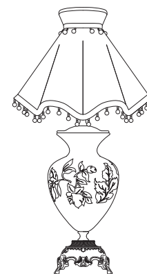
Art. 1587/P H 65 cm Pø 40 cm 1 x E27 X 40 W
