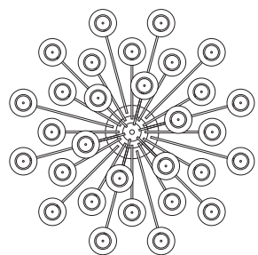
Art. 1447/CH30 H 90 cm ø 142 cm Po 16 cm 30 x E14 X 40W
