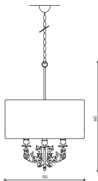
Art. 1461/CH3/BI H 60 cm Po 50 cm 3 x E14 X 60W
