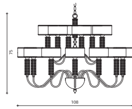
Art. 1423/CH18 H 75 cm ø 108 cm Pø 18 cm 18 x E14 X 40W
